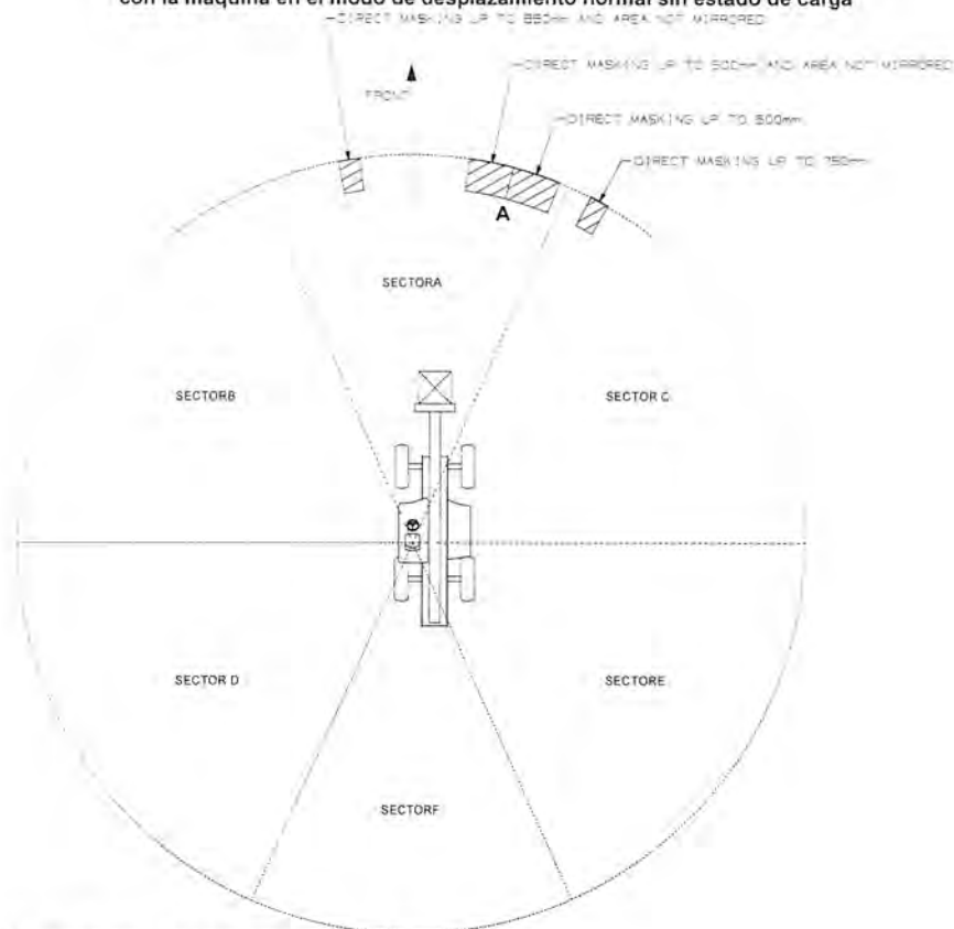
Figura 316. Ocultación de visibilidad en sectores A y C en la radio de 12 m, con la máquina en el modo de desplazamiento normal sin estado de carga
