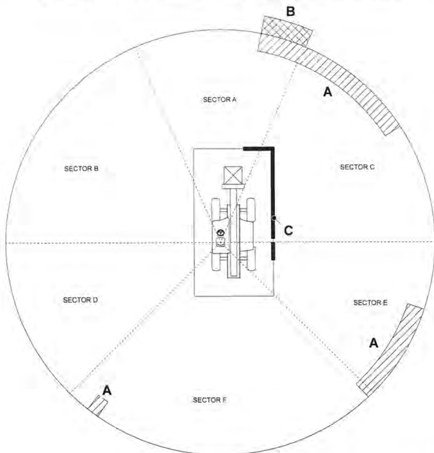
Figura 303. Ocultación de visibilidad en estado de carga de remolque del camión
