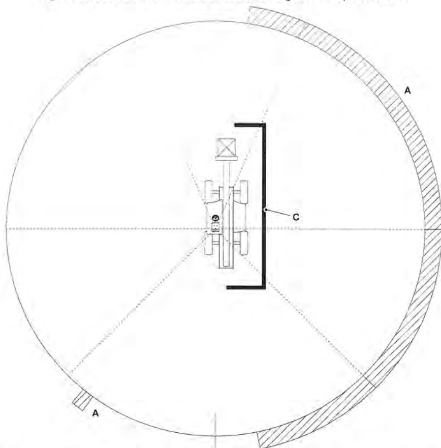
Figura 320. Ocultación de visibilidad en estado de carga de remolque del camión
