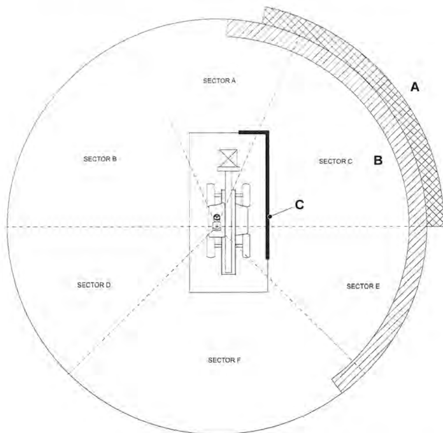
Figura 306. Ocultación de visibilidad en estado de carga de remolque del camión
