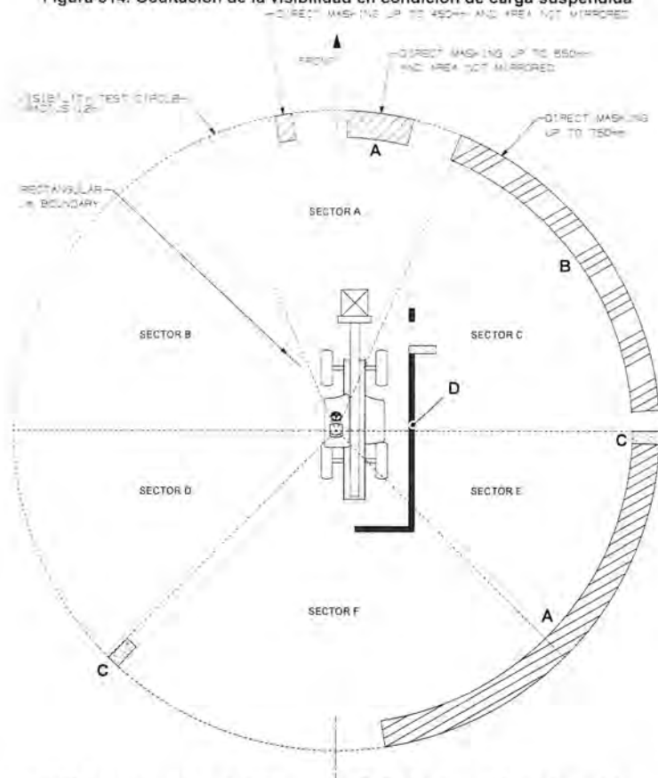
Figura 314. Ocultación de la visibilidad en condición de carga suspendida
