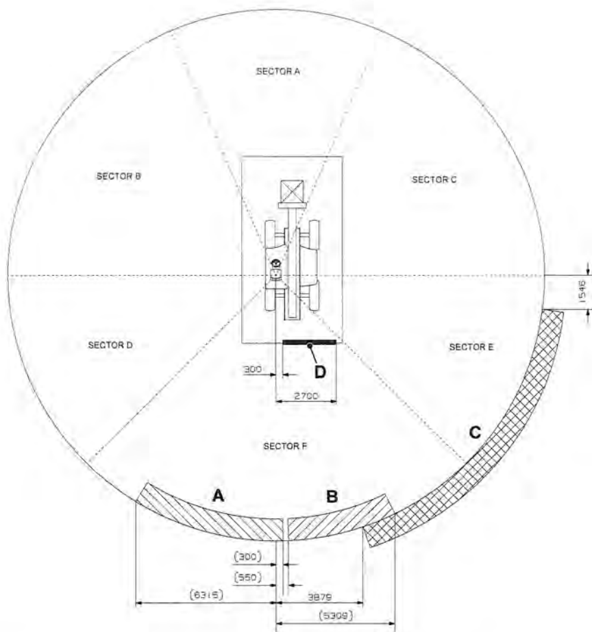
Figura 301. Ajuste del retrovisor
