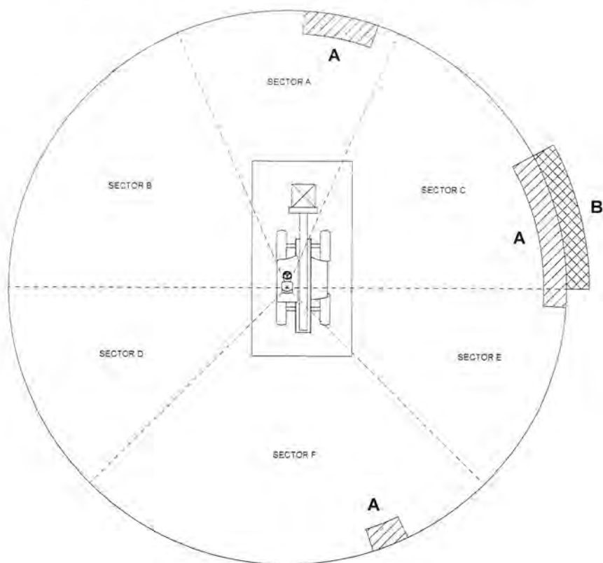
Figura 311. Ocultación de la visibilidad en condición de carga suspendida
