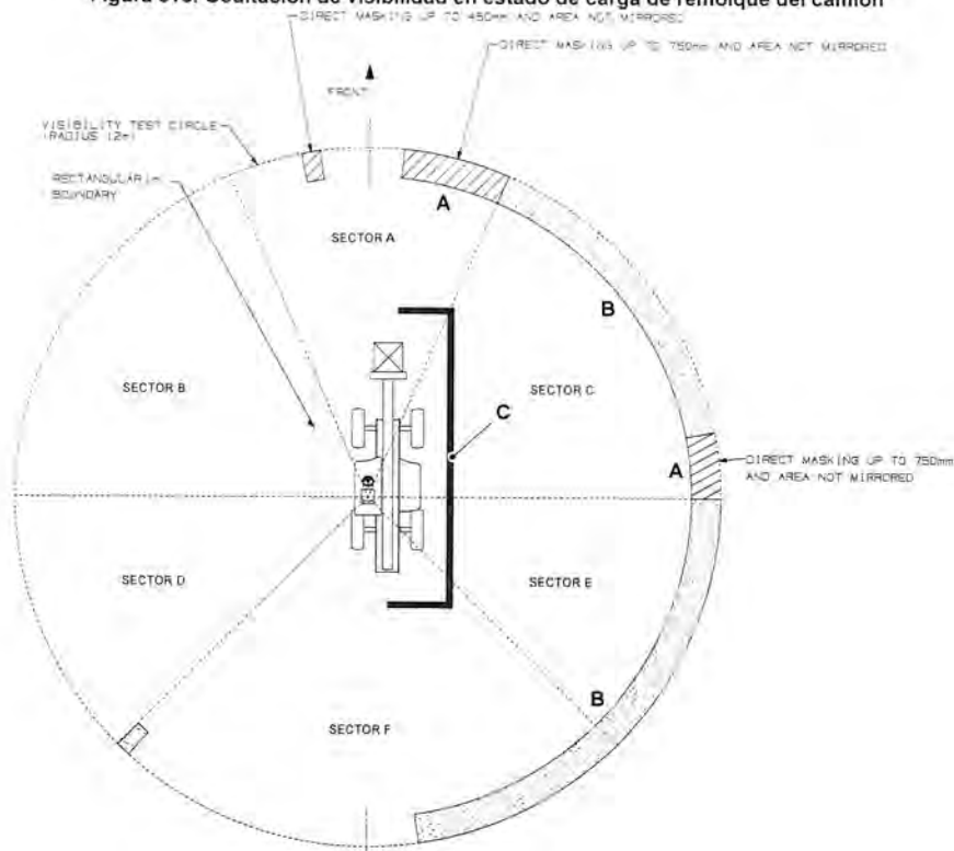
Figura 315. Ocultación de visibilidad en estado de carga de remolque del camión
