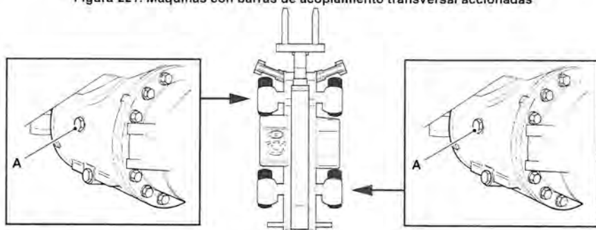
Figura 221. Máquinas con barras de acoplamiento transversal accionadas
