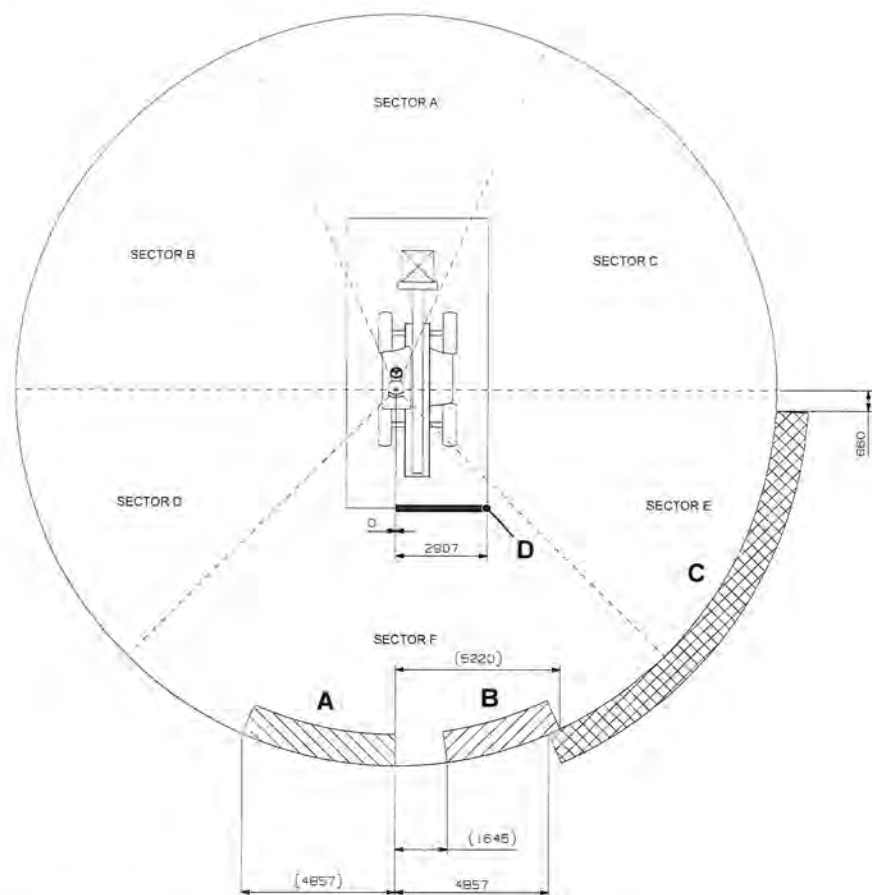
Figura 304. Ajuste del retrovisor
