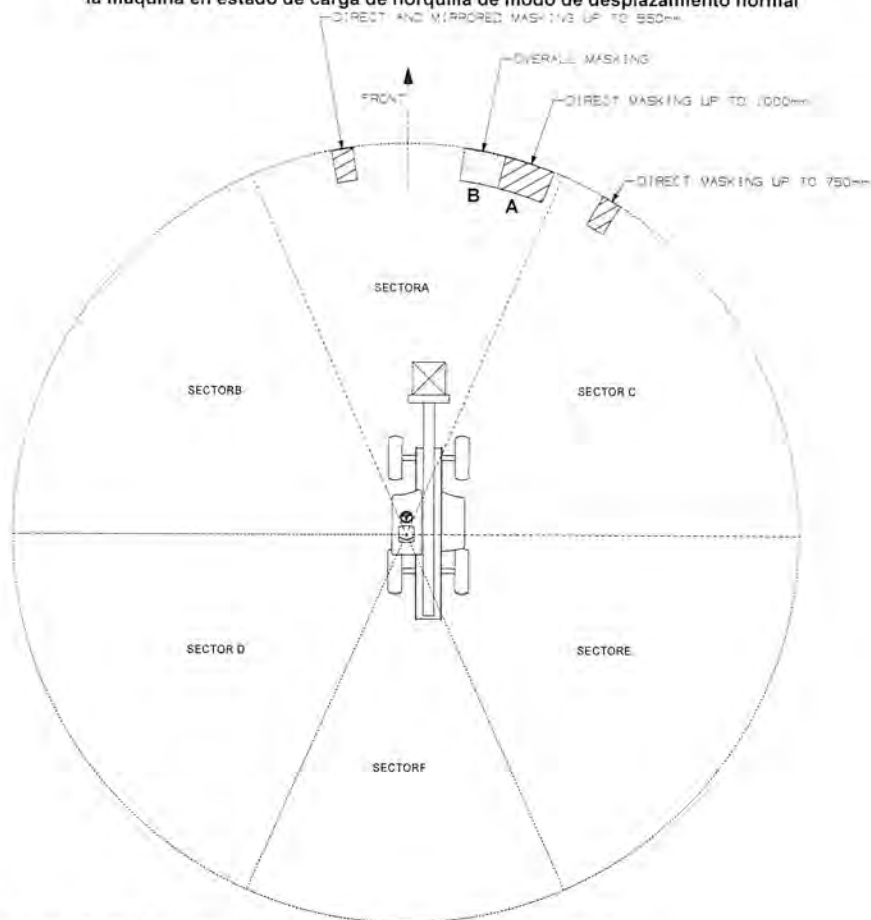
Figura 317. Ocultación de visibilidad en sectores A y C en el radio de 12 m, con la máquina en estado de carga de horquilla de modo de desplazamiento normal
