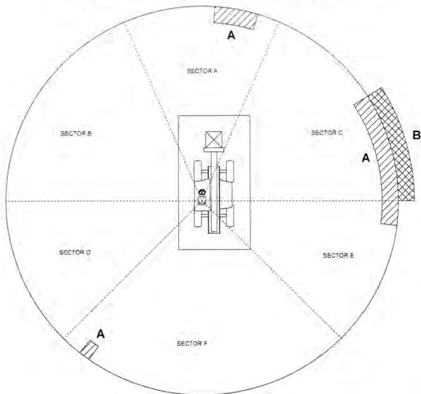
Figura 299. Ocultación de la visibilidad en condición de carga suspendida
