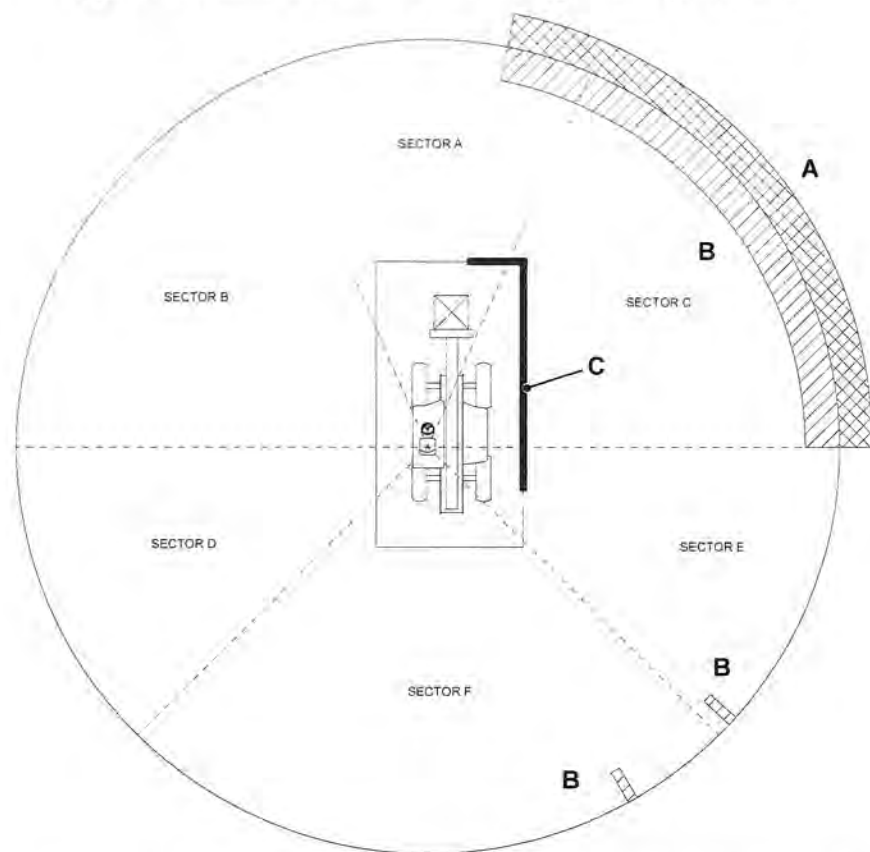
Figura 312. Ocultación de visibilidad en estado de carga de remolque del camión
