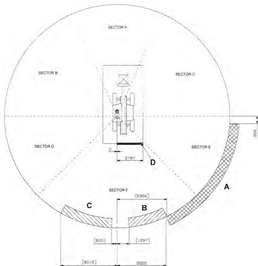
Figura 310. Ajuste del retrovisor
