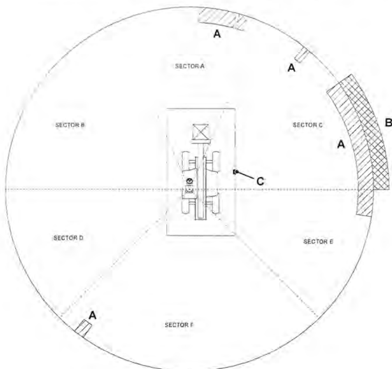
Figura 302. Ocultación de la visibilidad en condición de carga suspendida
