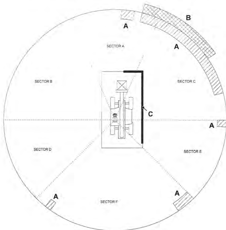
Figura 300. Ocultación de visibilidad en estado de carga de remolque del camión
