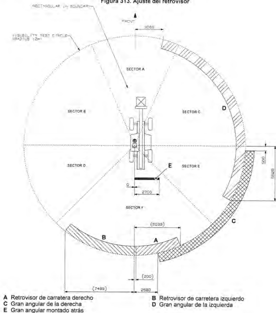
Figura 313. Ajuste del retrovisor
