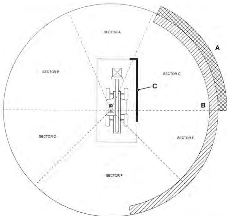
Figura 309. Ocultación de visibilidad en estado de carga de remolque del camión
