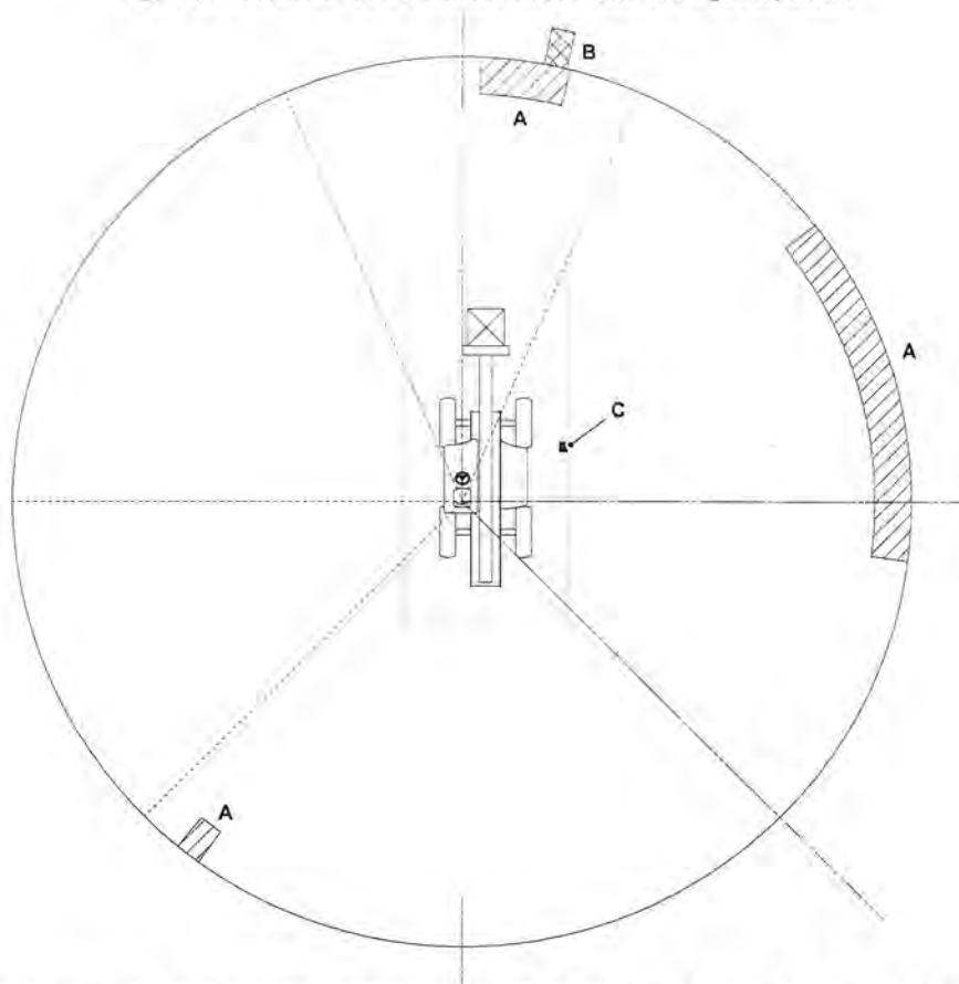
Figura 319. Ocultación de la visibilidad en condición de carga suspendida
