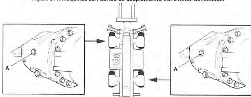
Figura 211. Máquinas con barras de acoplamiento transversal accionadas
