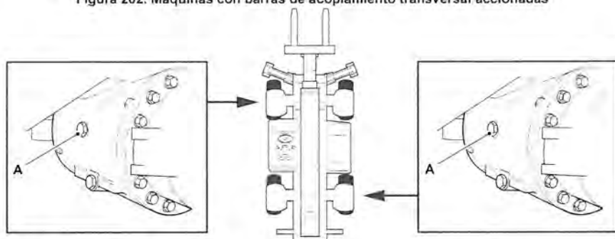
Figura 202. Máquinas con barras de acoplamiento transversal accionadas
